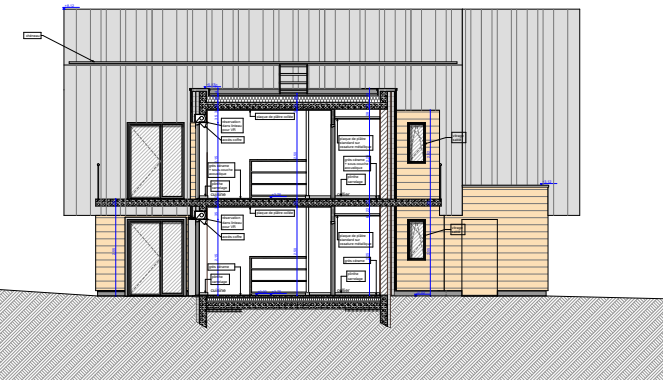
COUPE BB // éch. : 1/50"
