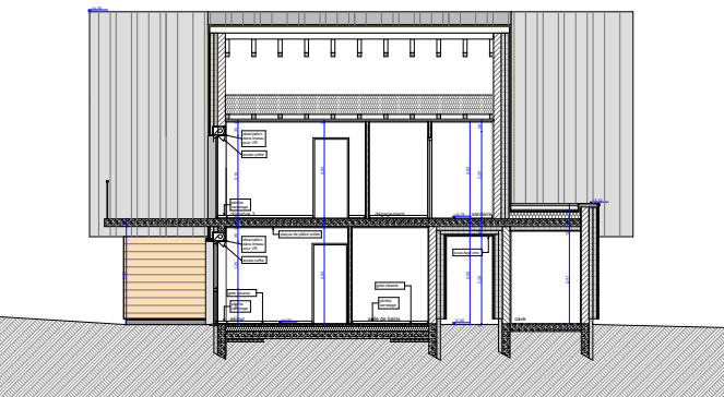
COUPE CC // éch. : 1/50"
