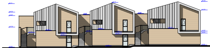
FAÇADES OUEST // éch. : 1/100"
