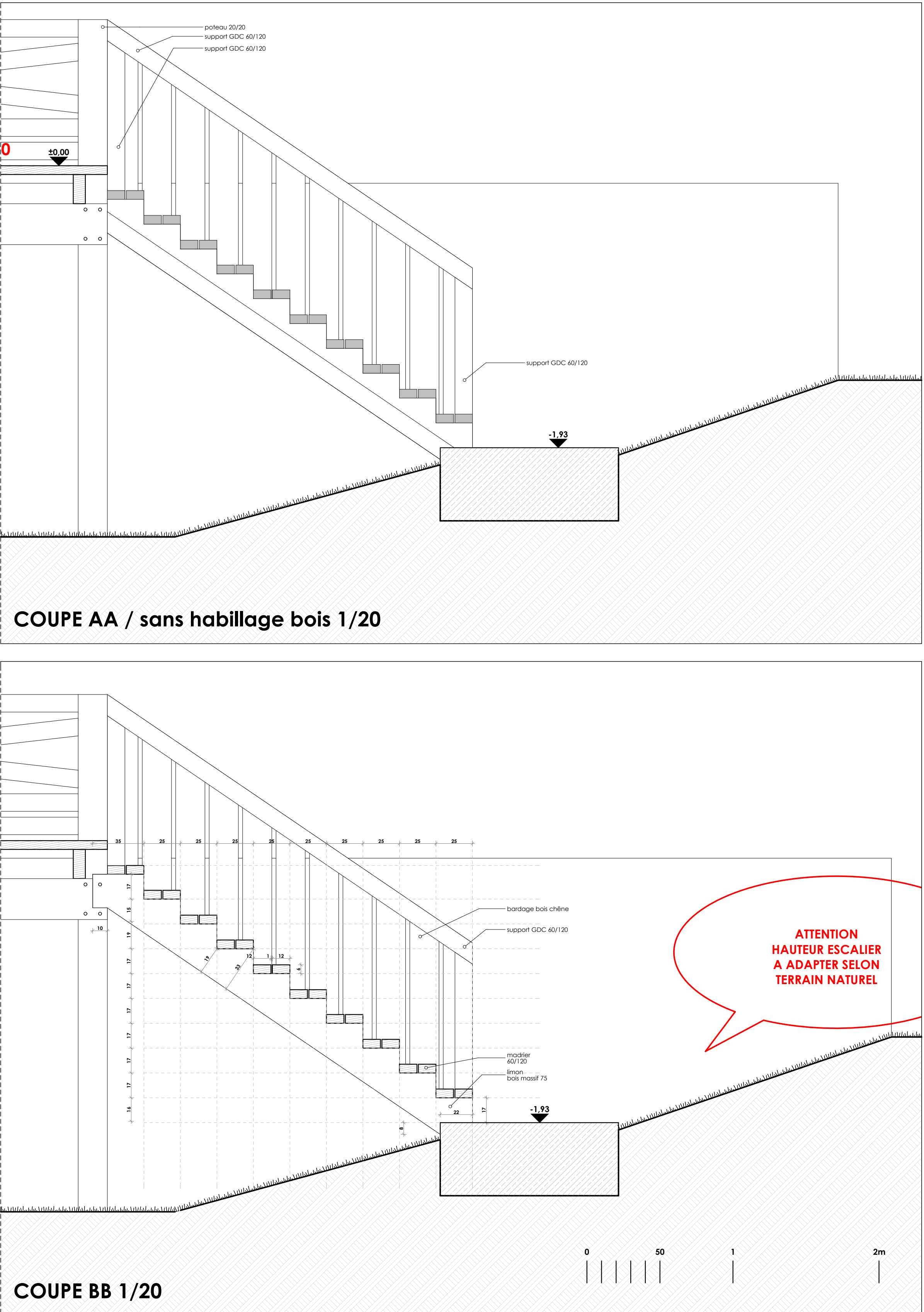
COUPE BB 1/20
