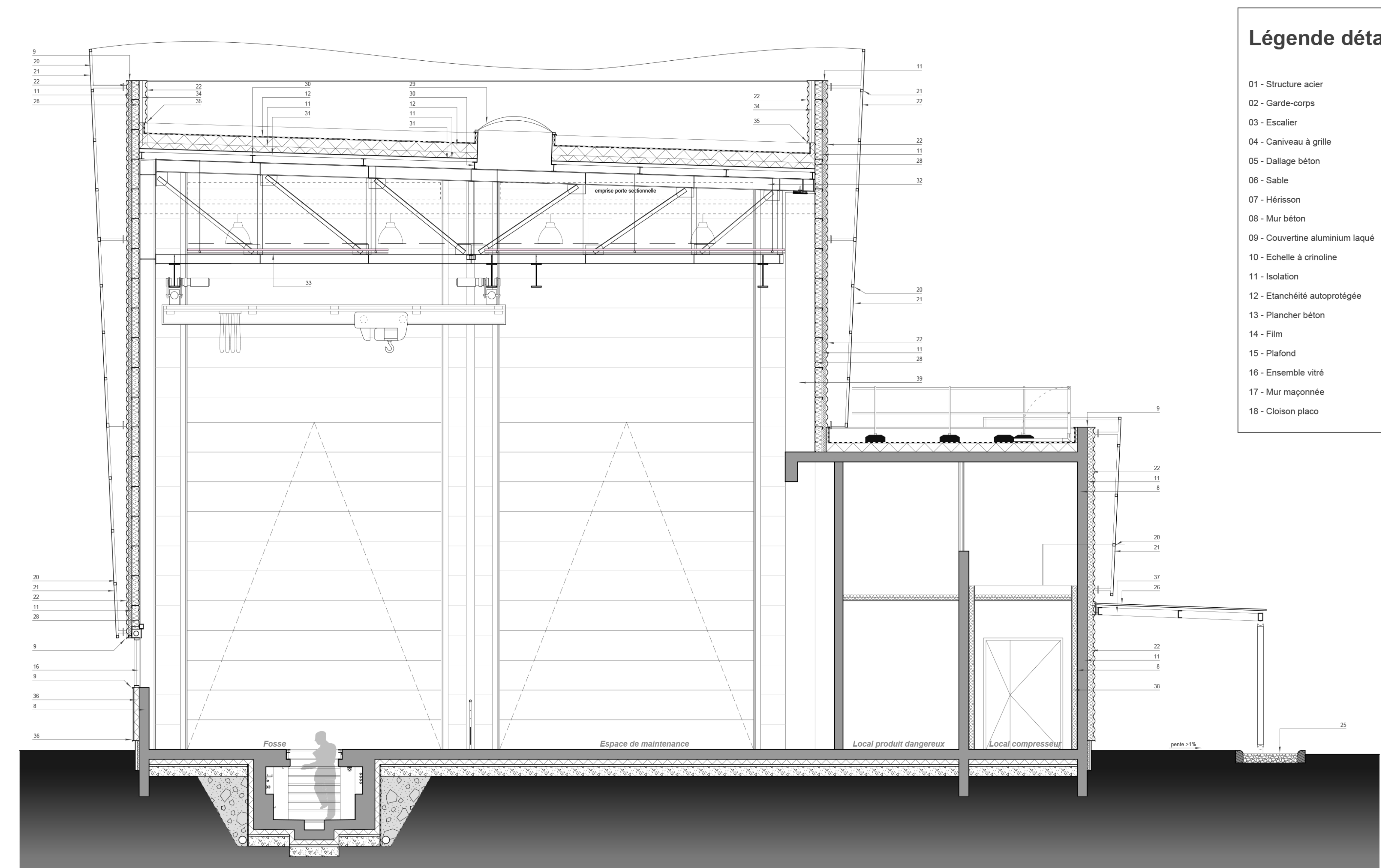
COUPE TRANSVERSALE BB 0 1 2 3 4 5 ECH : 1/50
