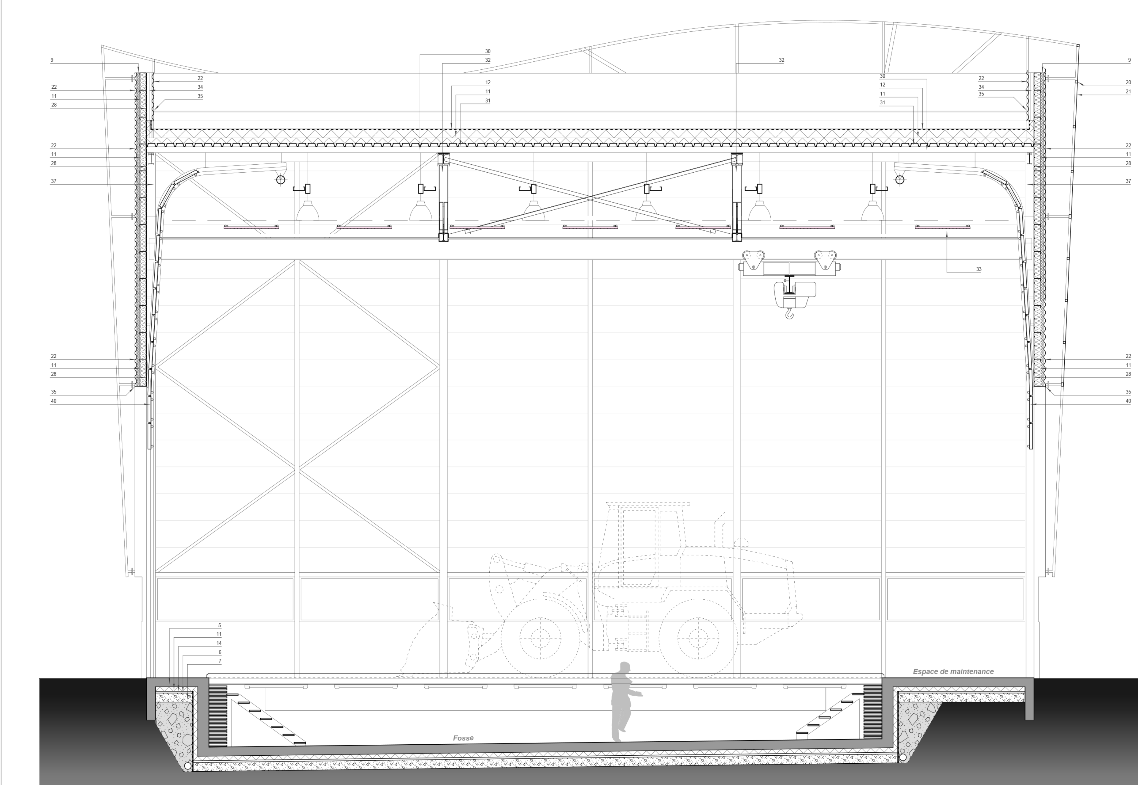
COUPE LONGITUDINALE AA 0 1 2 3 4 5 ECH : 1/50
