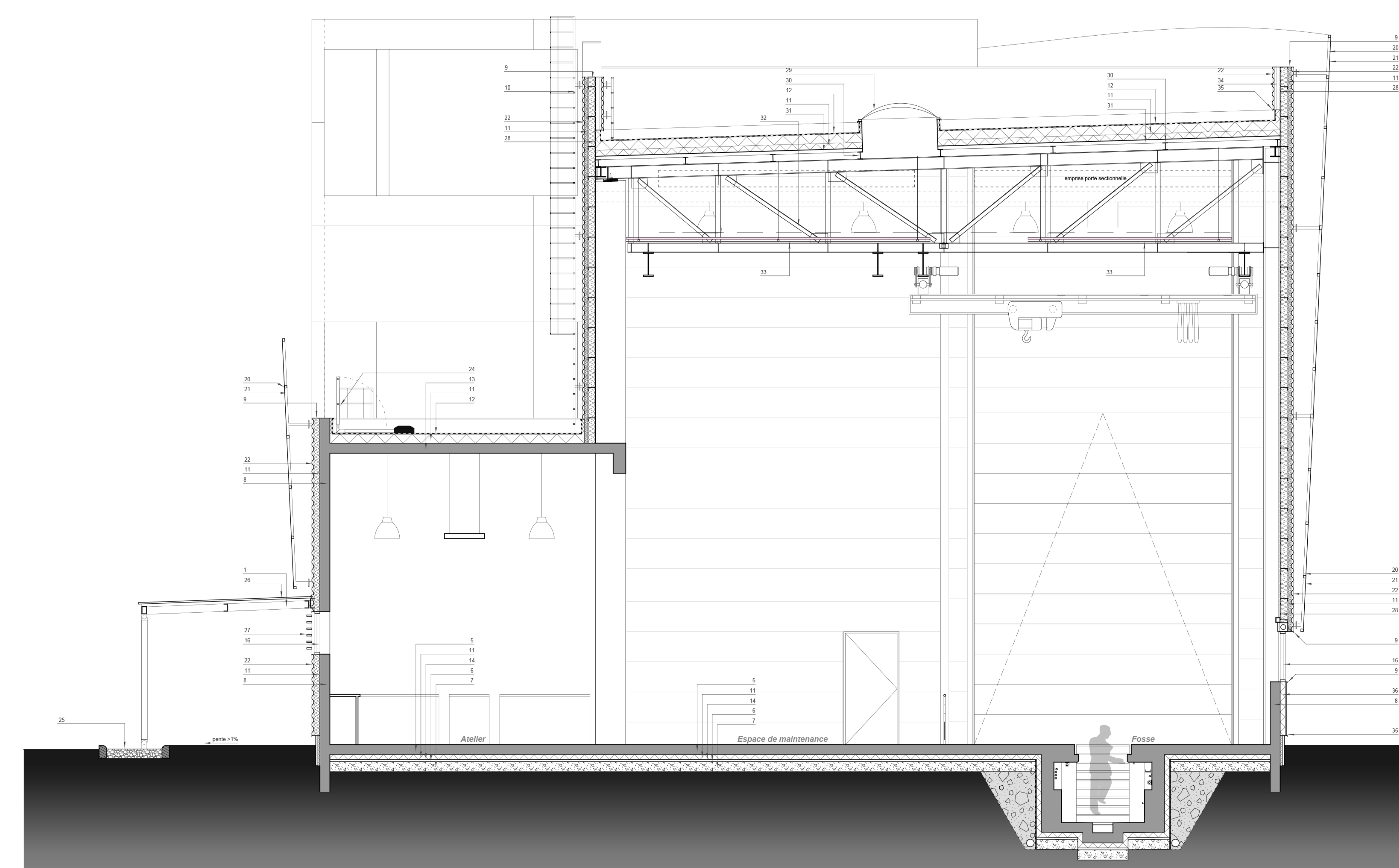
COUPE TRANSVERSALE DD 0 1 2 3 4 5 ECH : 1/50
