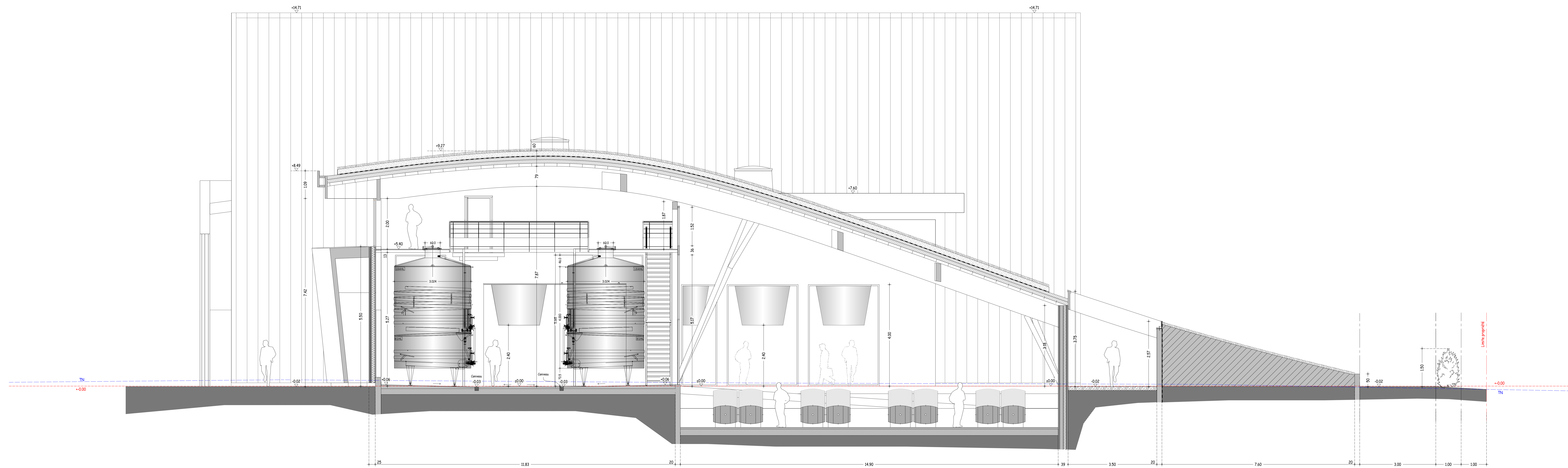
COUPE CC - ECHELLE : 1.50
