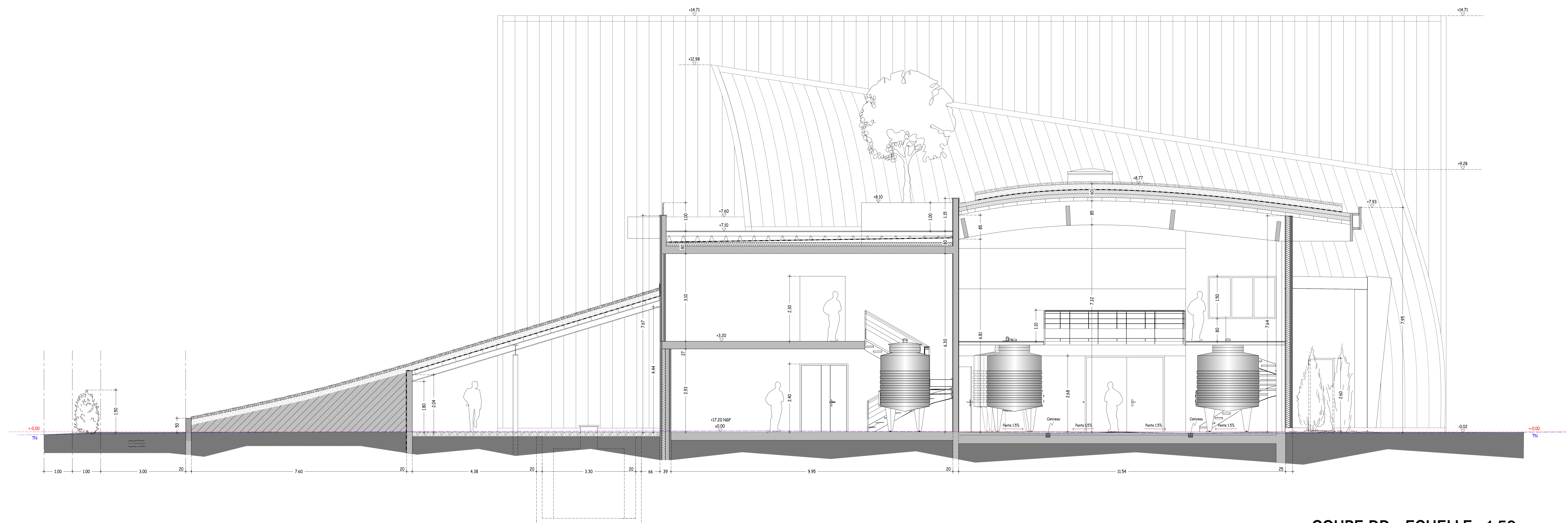
COUPE DD - ECHELLE : 1.50
