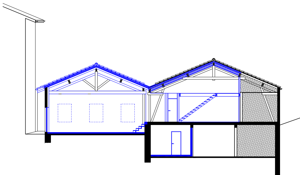
coupe transversale - état projet- 1:200 ème
