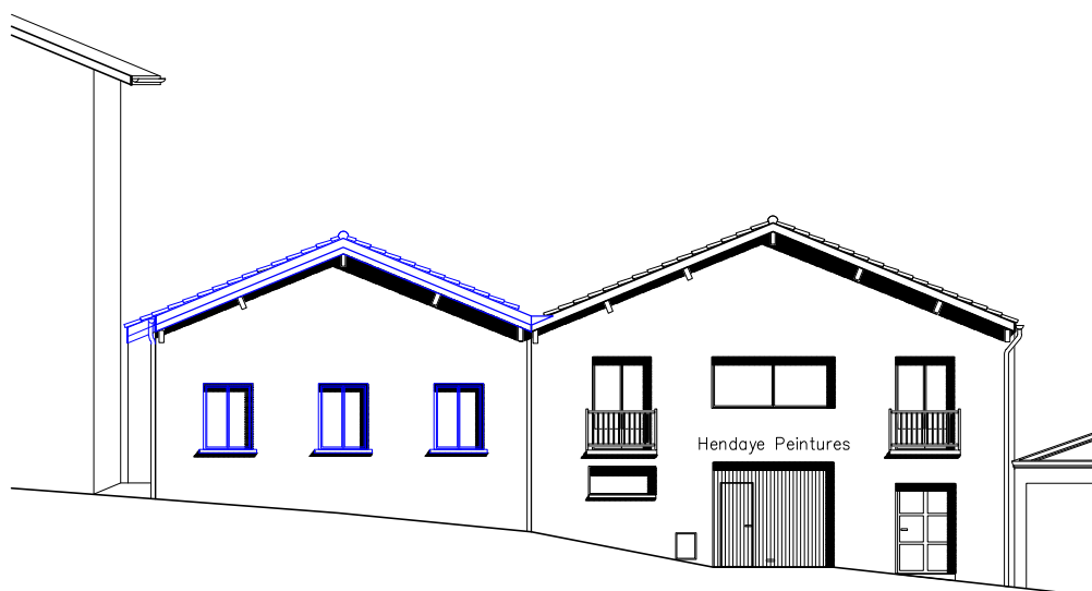
façade nord - état projet - 1:200 ème
