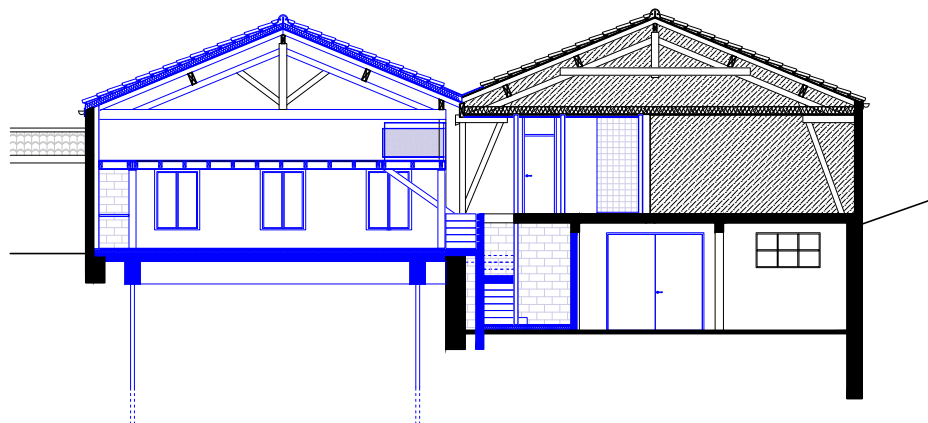
coupe transversale - état projet- 1:200 ème
