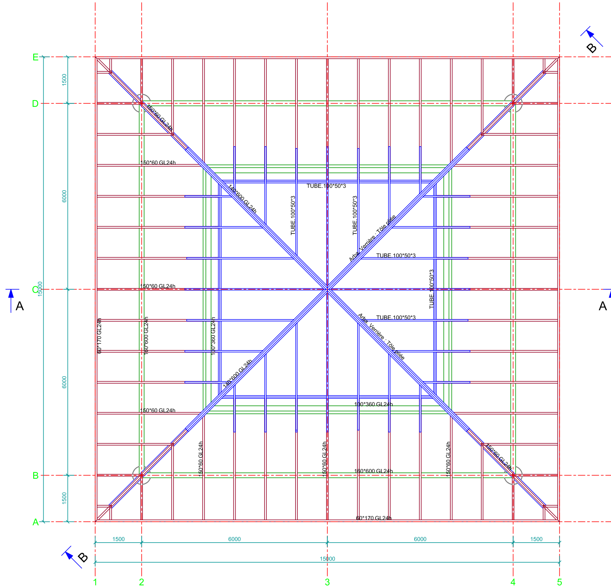
Vue en Plan 1:75
