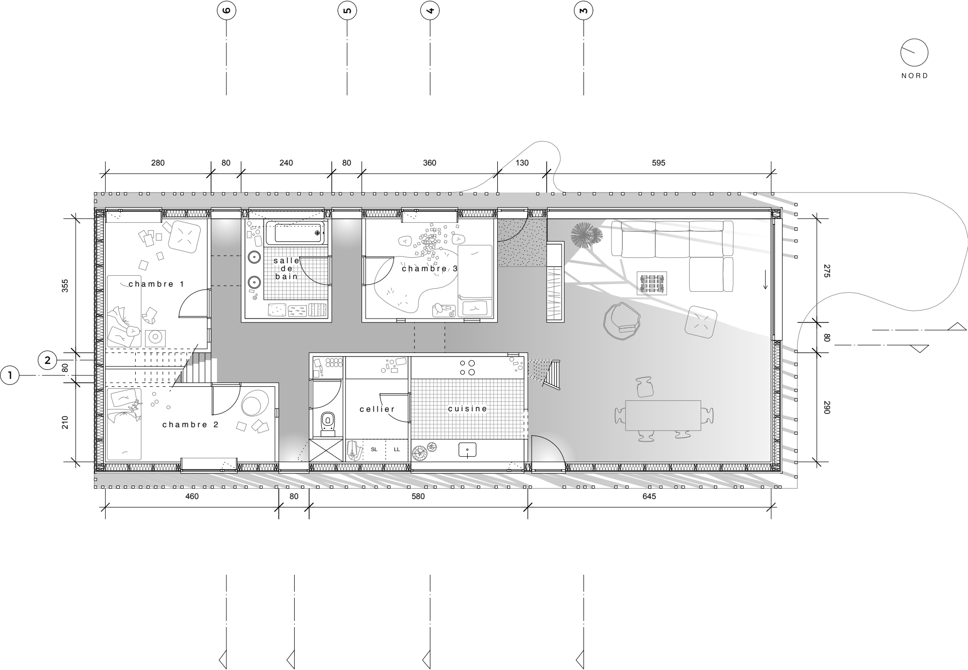
Plan niveau 0
